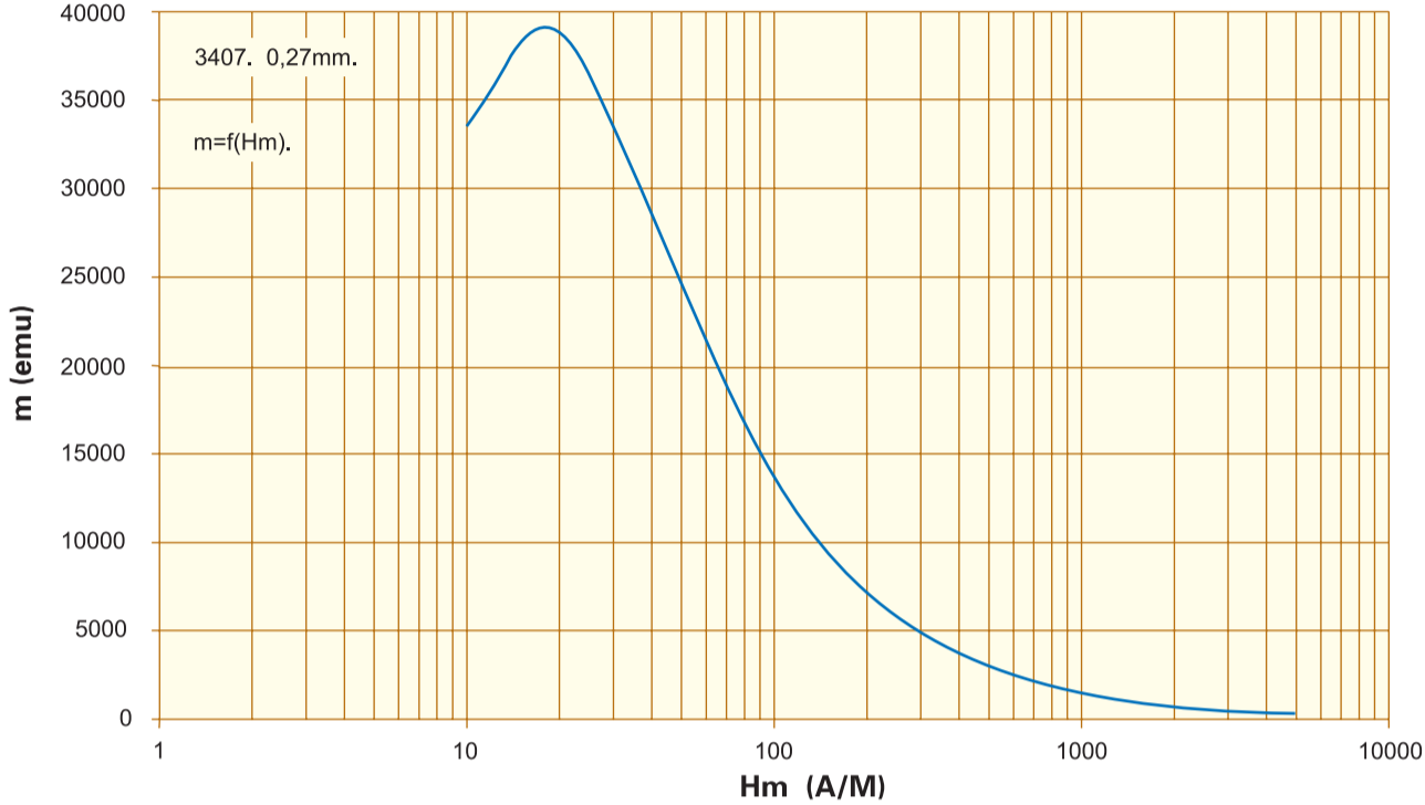
相对导磁率 Relative peak permeability. m=f(H_m) , F=50\text{Hz} . 0,27mm. 3407.
