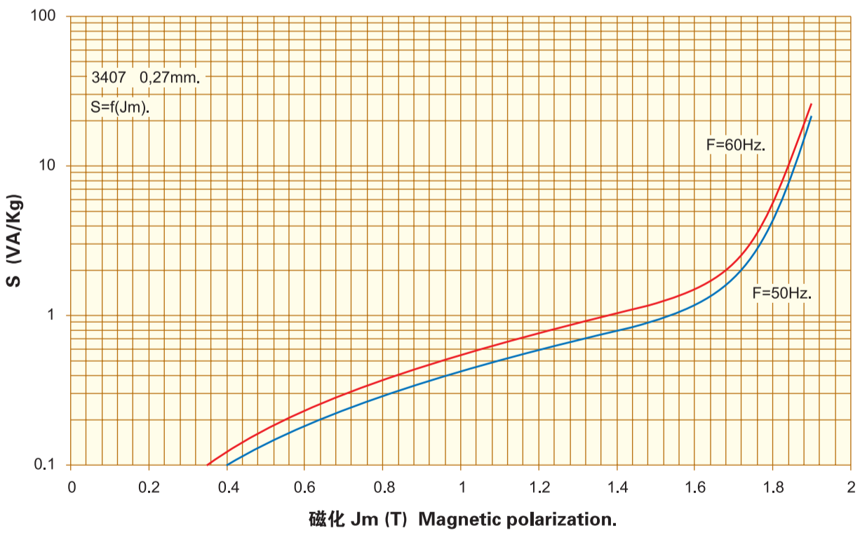
激磁功率. Exciting Power. S=f(J_m) 0,27mm. 3407
