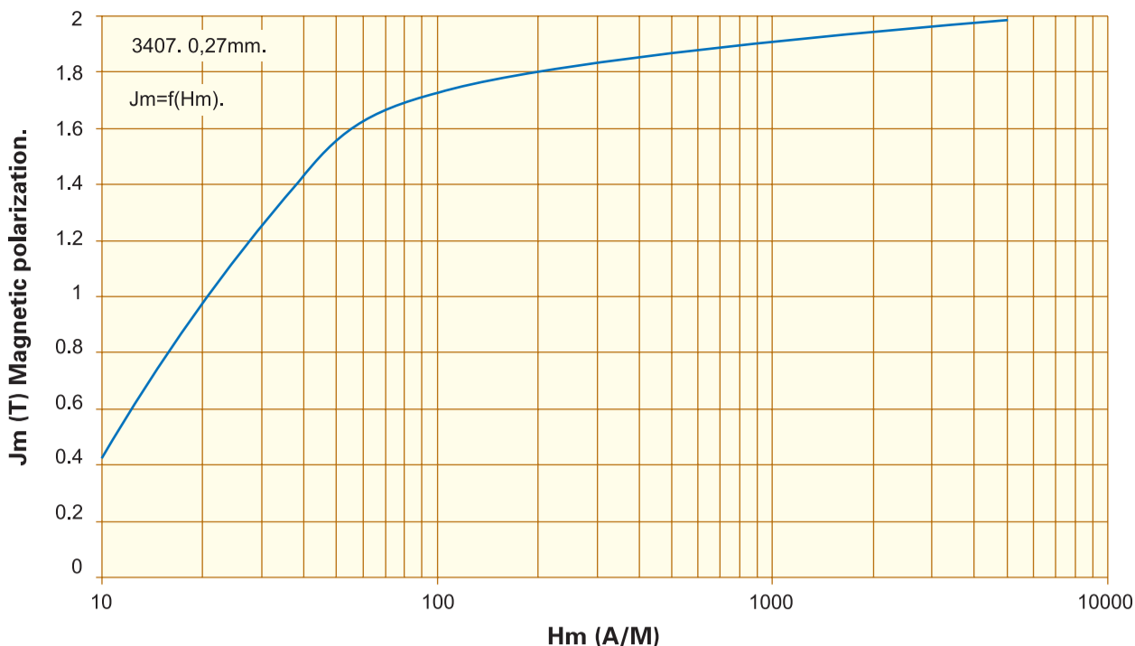
磁化曲线 Magnetic polarization. J_m=f(H_m) , F=50\text{Hz} . 0,27mm. 3407
