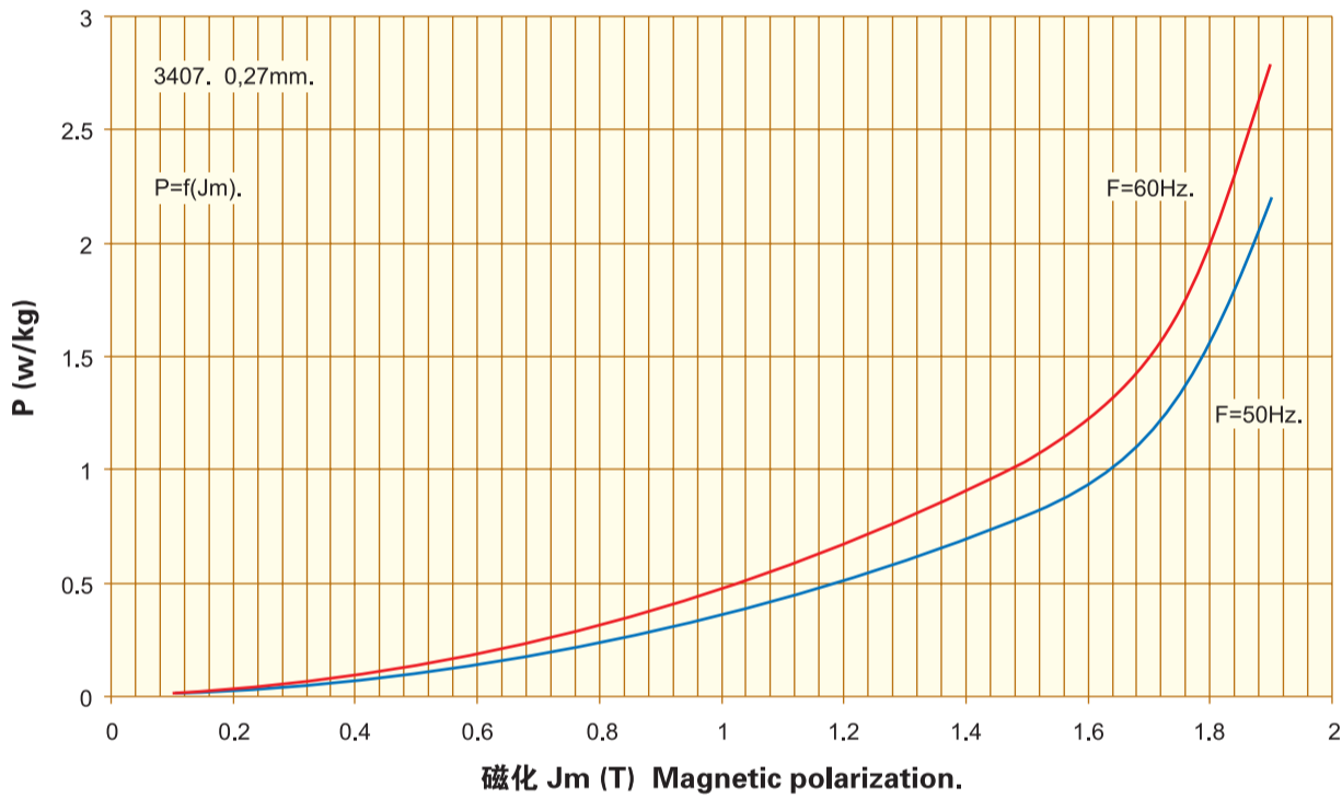
磁损耗. Specific Core Loss. P=f(J_m) 0,27mm. 3407
