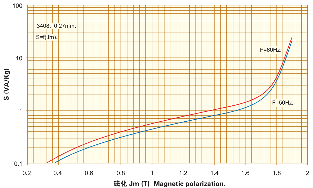
激磁功率. Exciting Power. S=f(J_m) 0,27mm. 3408
