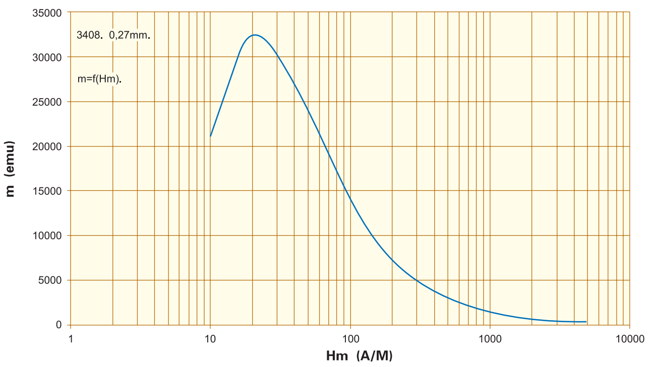
相对导磁率 Relative peak permeability. m=f(H_m) F=50\text{Hz} . 0,27mm. 3408.
