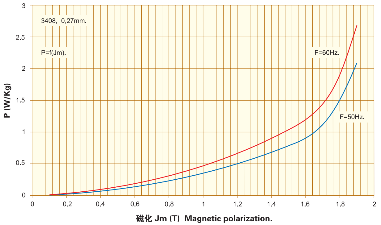
磁损耗 Specific Core Loss. P=f(J_m) , 0,27mm. 3408
