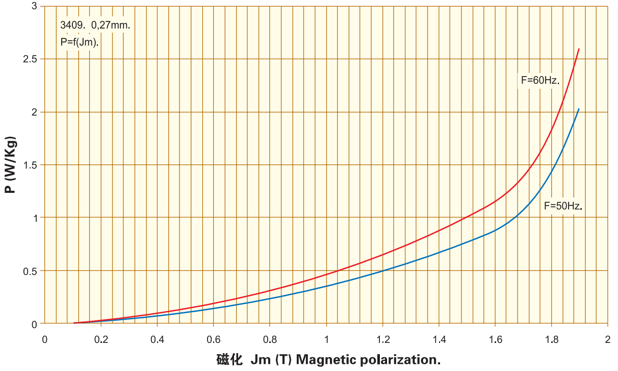
磁损耗 Specific Core Loss. P=f(J_m) , 0,27mm. 3409
